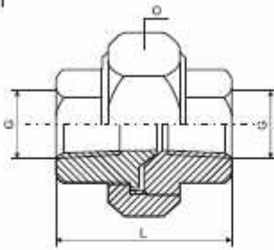
Śrubunek FF-NPT 3000 LBS
